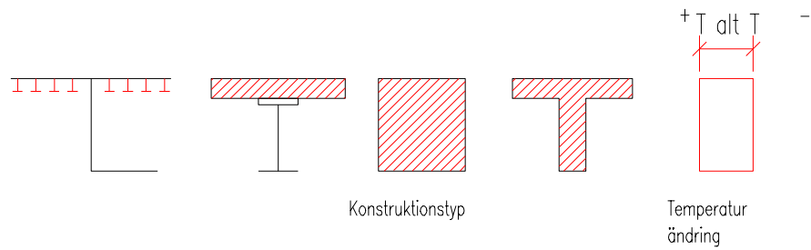
Figur 21-10 Jämn temperaturändring
