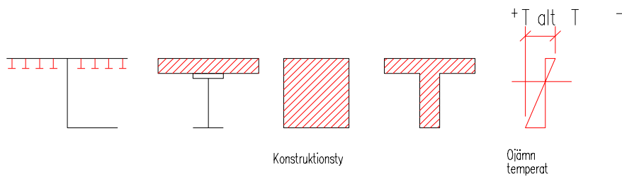
Figur 21-11 Ojämn temperaturändring
