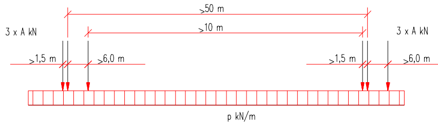
Figur 21-4 Ekvivalentlast typ 5
