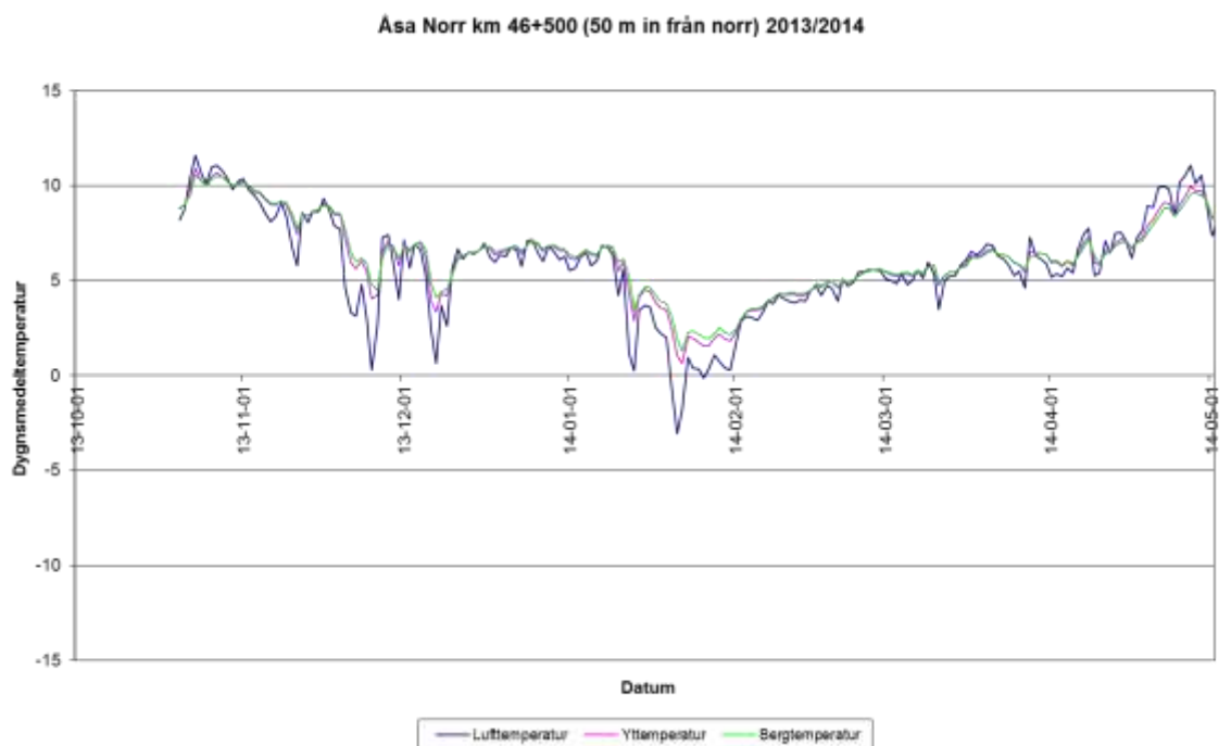
Figur 6 Luft-, yt- och bergtemperatur vid 50 m in från norra mynningen under perioden 2013-10-01 till 2014-05-01
