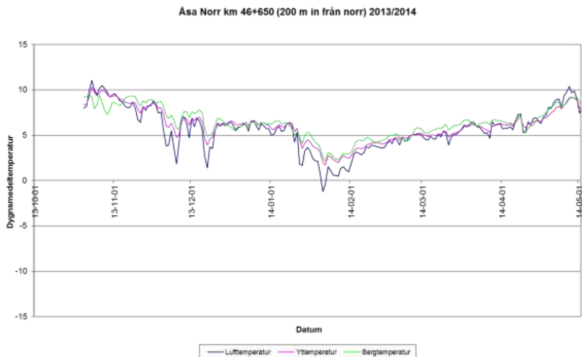
Figur 8 Luft-, yt- och bergtemperatur vid 200 m in från norra mynningen under perioden 2013-10-01 till 2014-05-01
