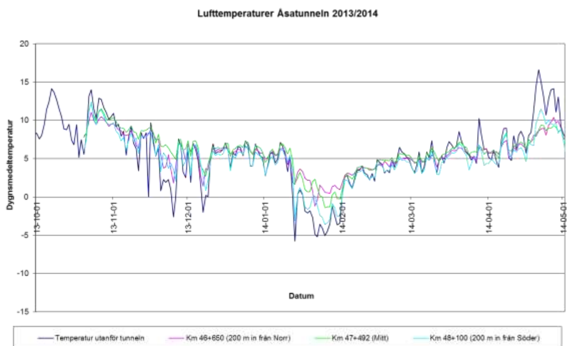
Figur 4 Lufttemperaturer i och utanför Åsatunneln från 2013-10-01 till 2014-05-01
