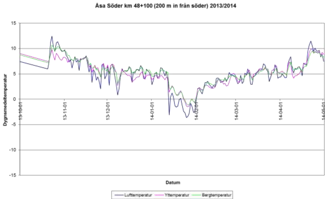
Figur 12 Luft-, yt- och bergtemperatur vid 200 m in från södra mynningen under perioden 2013-10-01 till 2014-05-01
