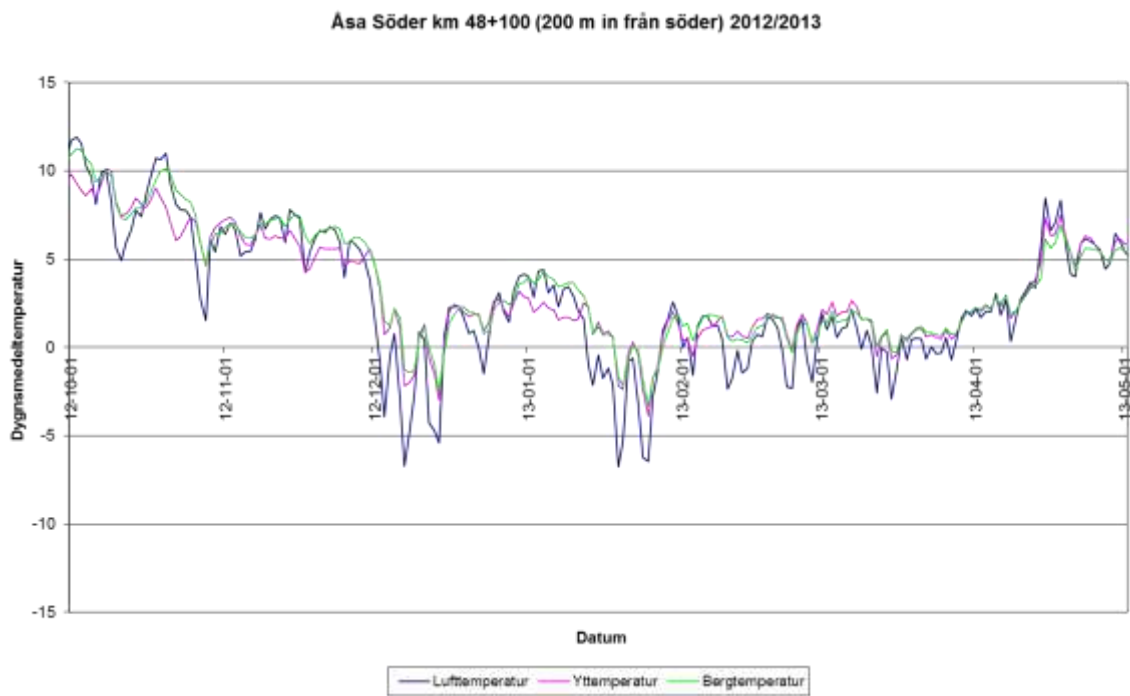
Figur 11 Luft-, yt- och bergtemperatur vid 200 m in från södra mynningen under perioden 2012-10-01 till 2013-05-01
