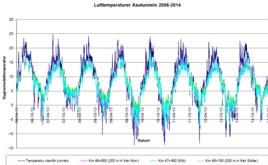
Figur 1 Lufttemperaturer i och utanför Åsatunneln från 2006-04-13 till 2014-05-01
