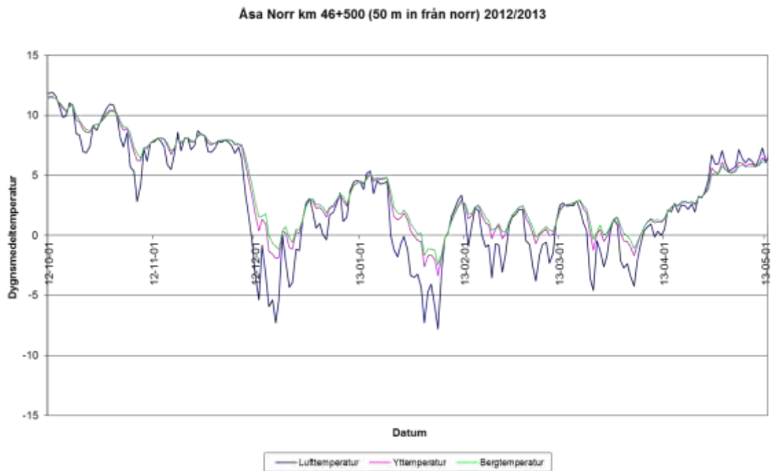
Figur 5 Luft-, yt- och bergtemperatur vid 50 m in från norra mynningen under perioden 2012-10-01 till 2013-05-01
