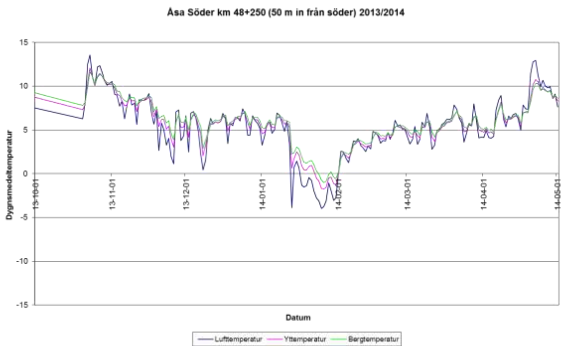
Figur 14 Luft-, yt- och bergtemperatur vid 50 m in från södra mynningen under perioden 2013-10-01 till 2014-05-01
