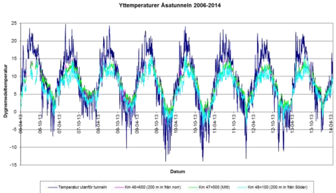
Figur 2 Yttemperaturer i Åsatunneln från 2006-04-13 till 2014-05-01
