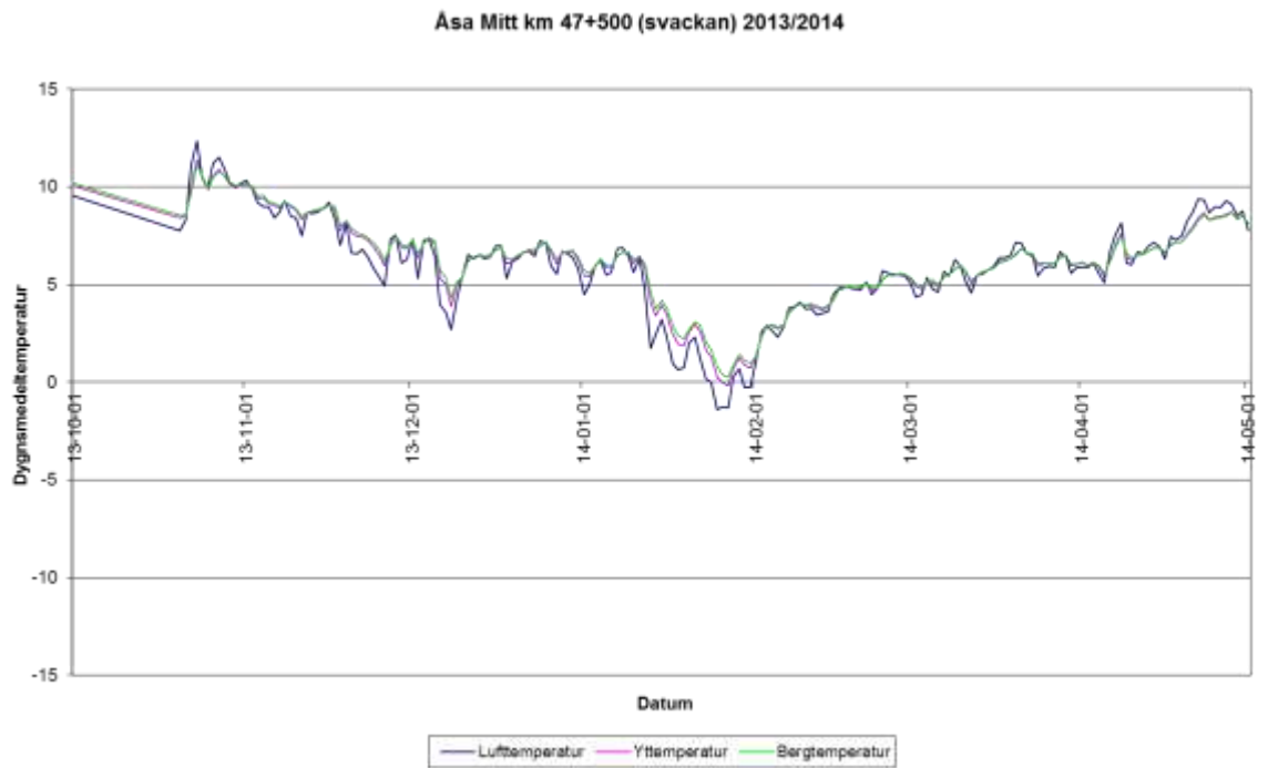
Figur 10 Luft-, yt- och bergtemperatur vid svackan i mitten av tunneln under perioden 2013-10-01 till 2014-05-01
