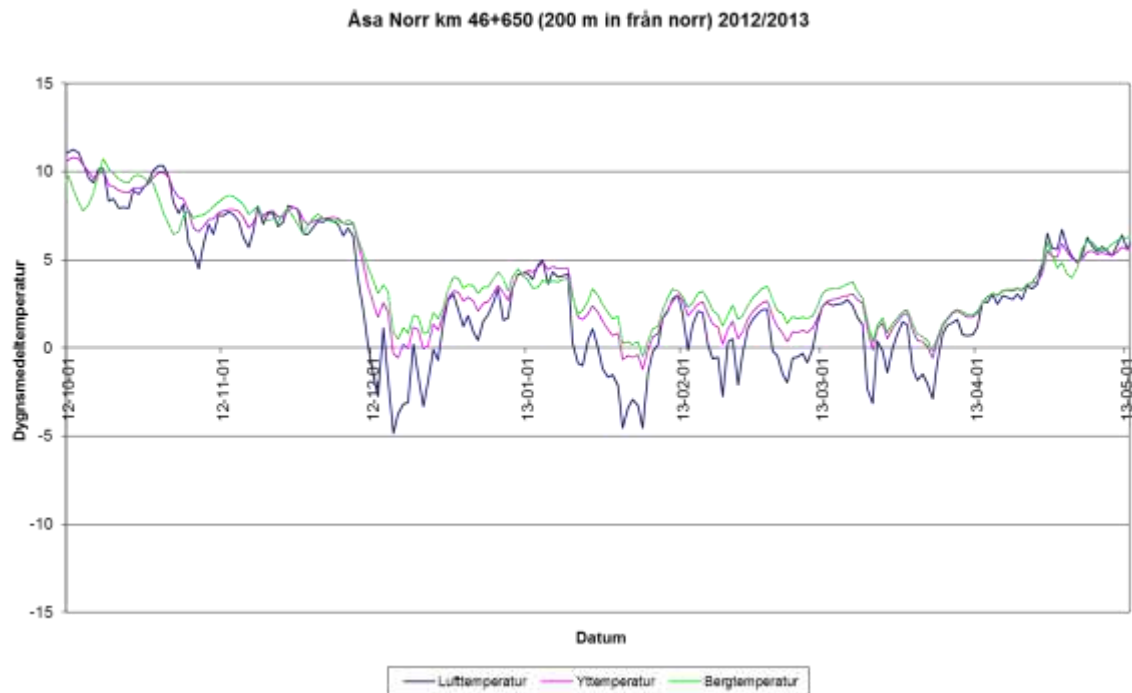
Figur 7 Luft-, yt- och bergtemperatur vid 200 m in från norra mynningen under perioden 2012-10-01 till 2013-05-01
