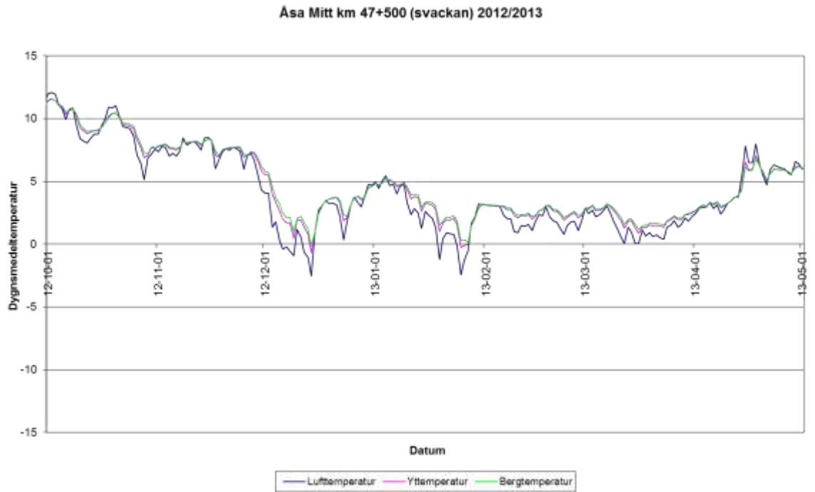
Figur 9 Luft-, yt- och bergtemperatur vid svackan i mitten av tunneln under perioden 2012-10-01 till 2013-05-01
