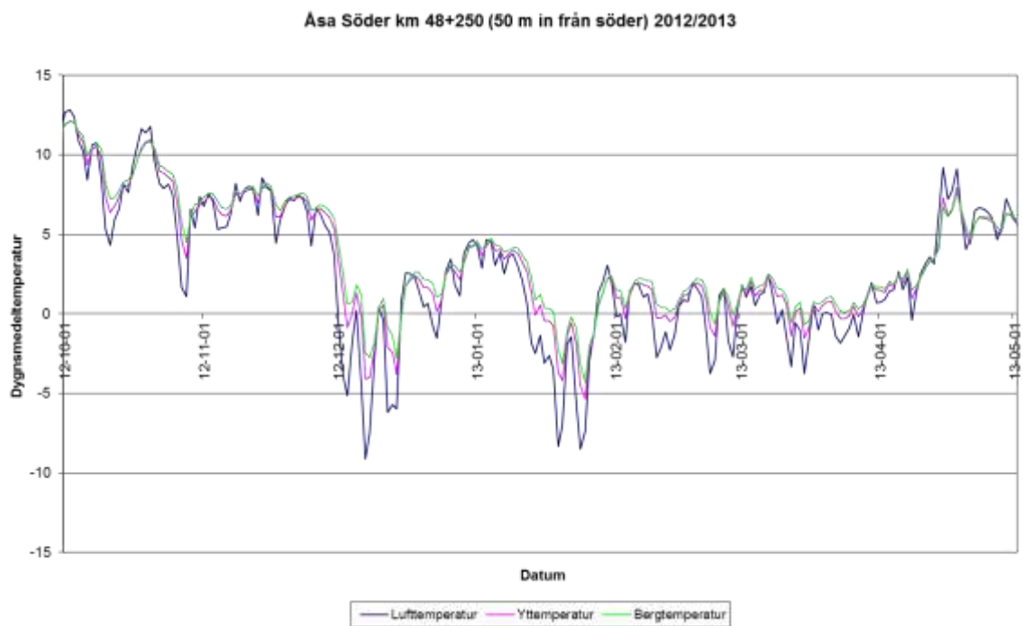
Figur 13 Luft-, yt- och bergtemperatur vid 50 m in från södra mynningen under perioden 2012-10-01 till 2013-05-01
