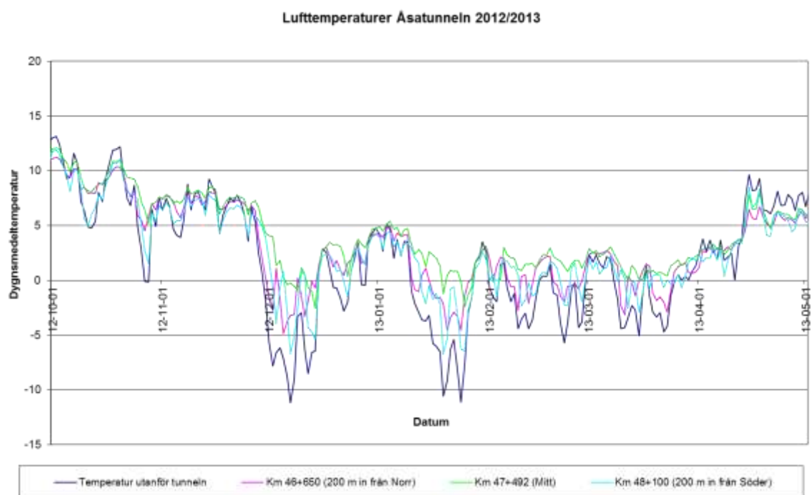
Figur 3 Lufttemperaturer i och utanför Åsatunneln från 2012-10-01 till 2013-05-01
