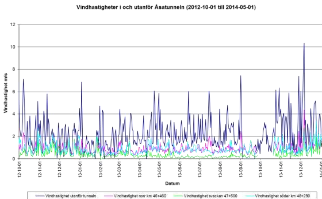
Figur 15 Vindhastighet i och utanför tunneln under perioden 2012-10-01 till 2014-05-01
